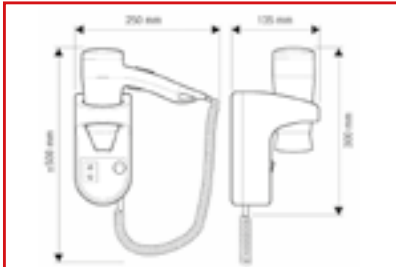
PREMIUM SMART & ACTION SHAVER 301000 / 301100 / 301200 / 300805 / 300809 / 301001
